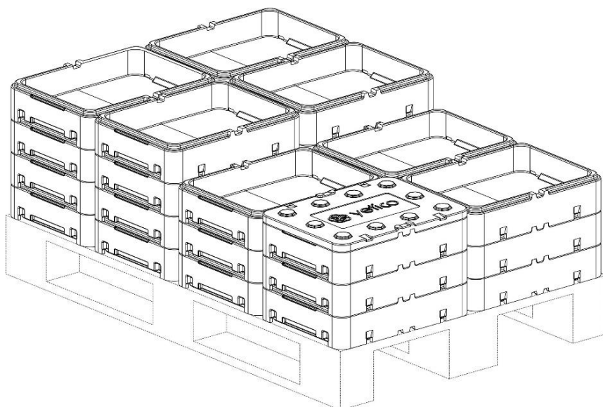
AUFSTELLVORSCHLAG DER WEBOX 400X300 VERPACKUNGEN AUF EINER EUROPALETTE (1200 X 800 MM).
